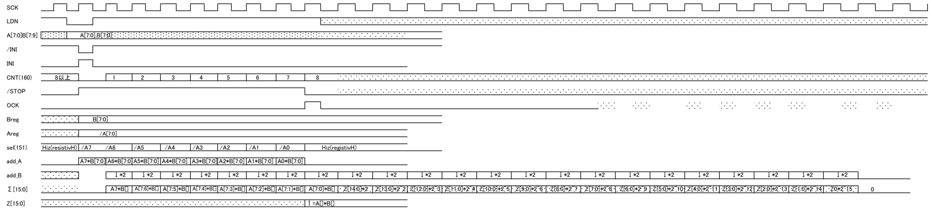
繰り返し加算型 乗算機(8bit * 8bit=16bit) 同期実行
